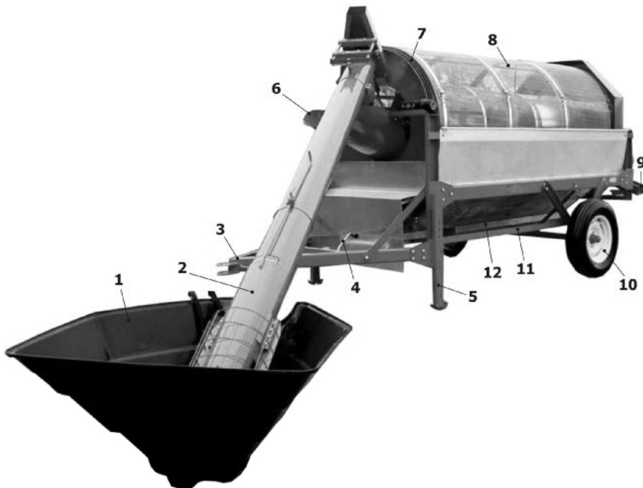
Рис. 1 Общий вид зерноочистителя
