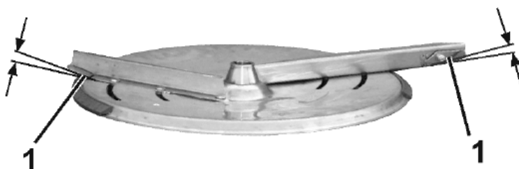
Рисунок 5.5 - Регулировка поворотных пластин
