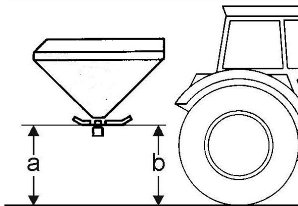
Рисунок 5.3 - Высота над поверхностью поля при стандартном удобрении
