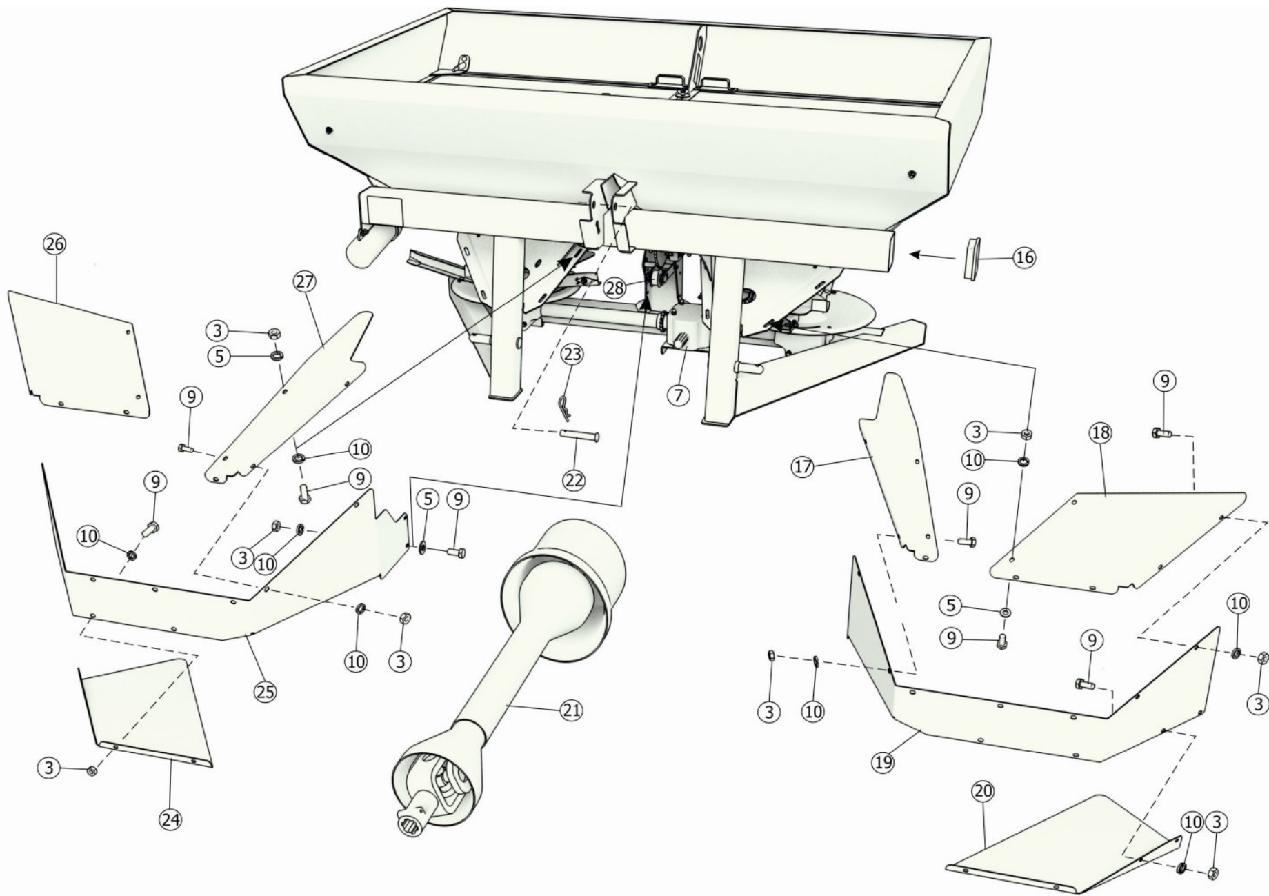
Рисунок 2 – Разбрасыватель PA-900.00.00.000. Общий вид
