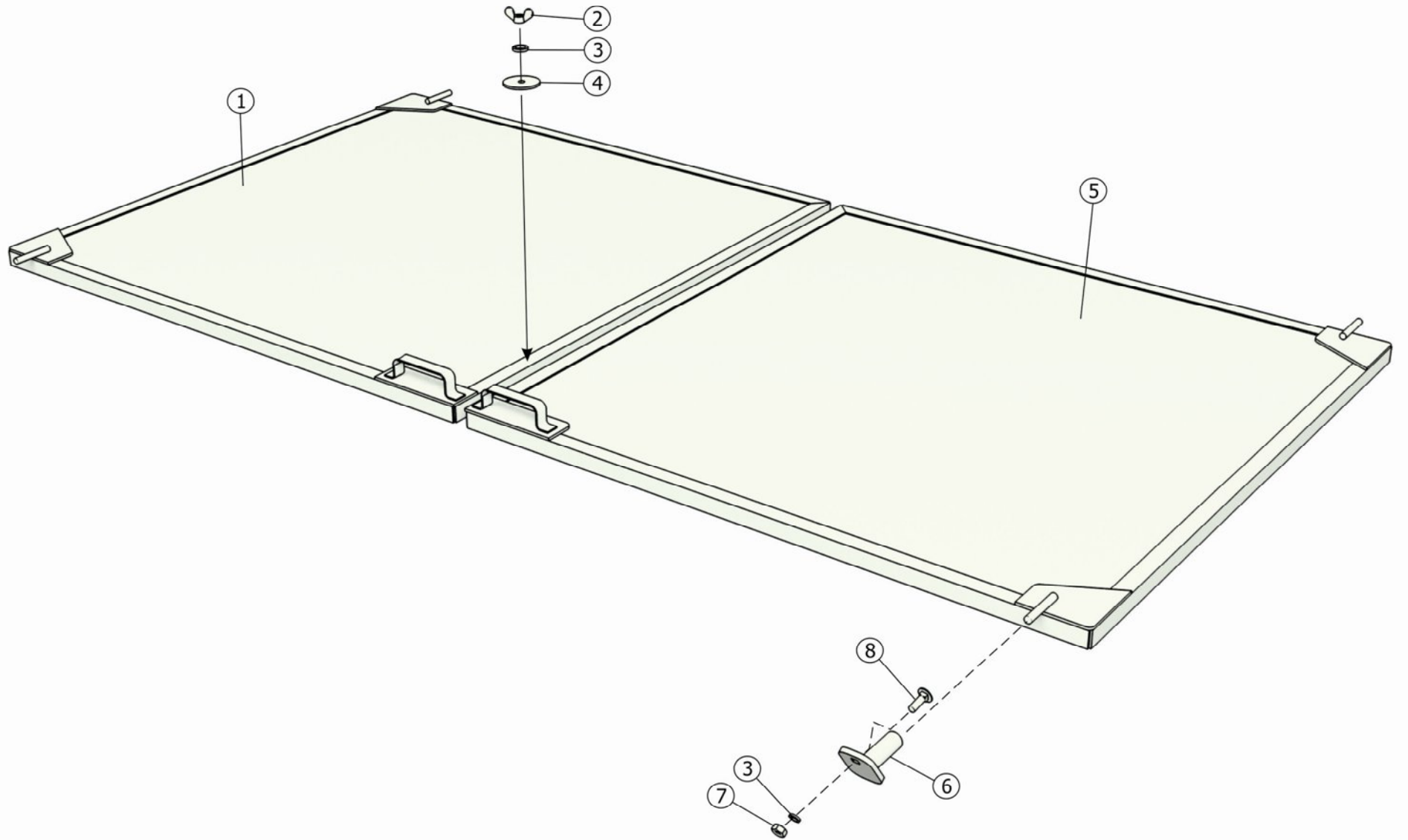
Рисунок 3 – Установка сетки PA-900.30.00.000A
