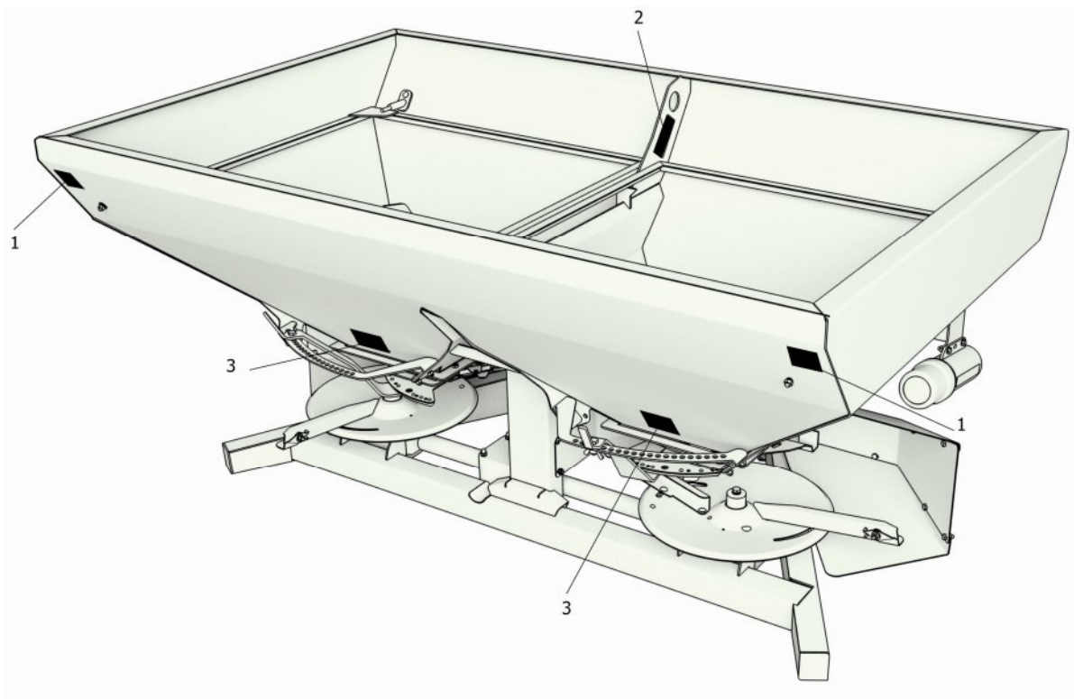
Рисунок 4.1 – Место расположения табличек
