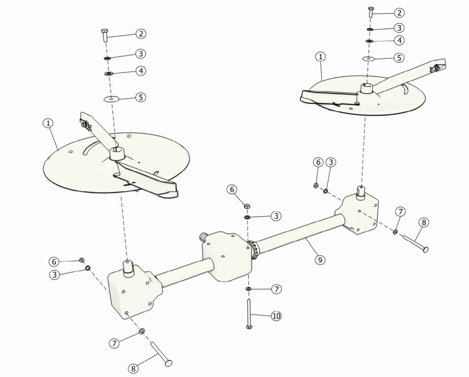
Рисунок 4 – Установка редуктора РА-900.70.000Б
