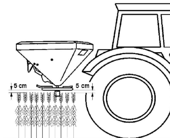
Рисунок 5.4 - Высота над поверхностью поля при позднем внесении удобрения
