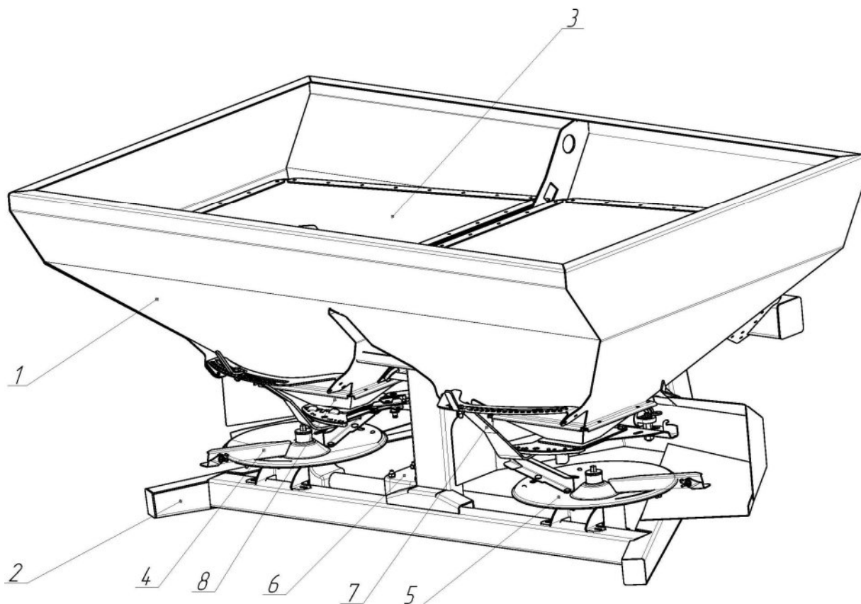
Рисунок 3.1- Общий вид разбрасывателя РА-900
