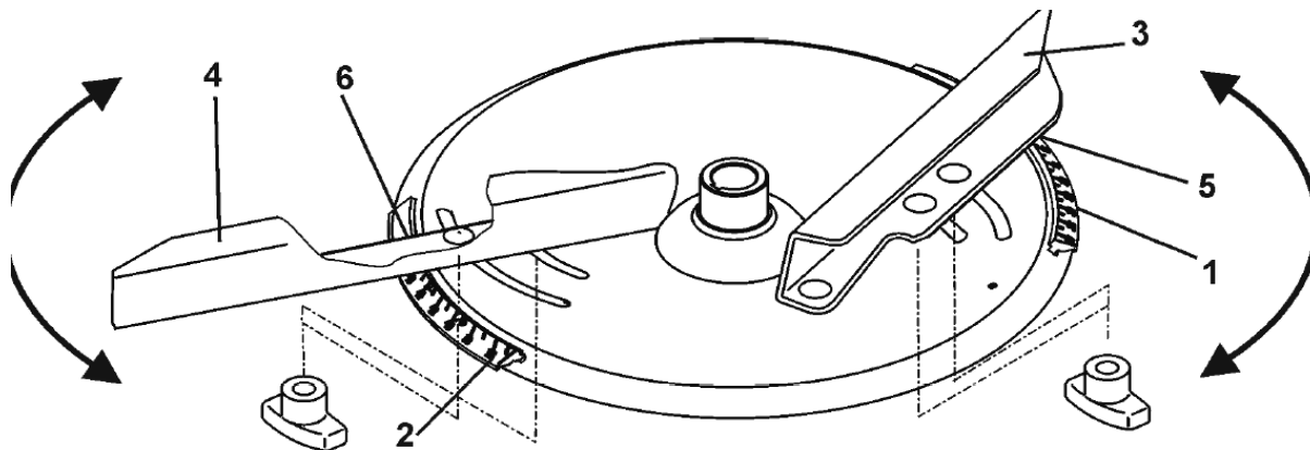
Рисунок 5.2- Распределяющий диск
